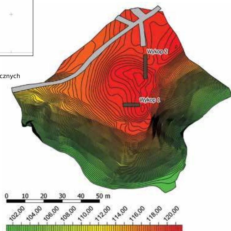
Ryc. 10. Plan sytuacyjno-wysokościowy grodziska w Zimnochach, st. 2 z rozmieszczeniem wykopów badawczych (na podstawie pomiarów J. Błaszczyka, oprac. R. Solecki)
