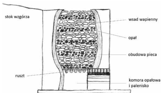
Ryc. 26. Rekonstrukcje wapienników okresowych (rys. K. Rabiega, wg: Smith 2011: 4)
