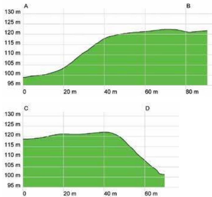
Ryc. 6. Przekroje przez grodziska w Zimnochach, st. 2 uzyskane z danych ALS (na podstawie materiałów CODGIK, oprac. R. Solecki)
