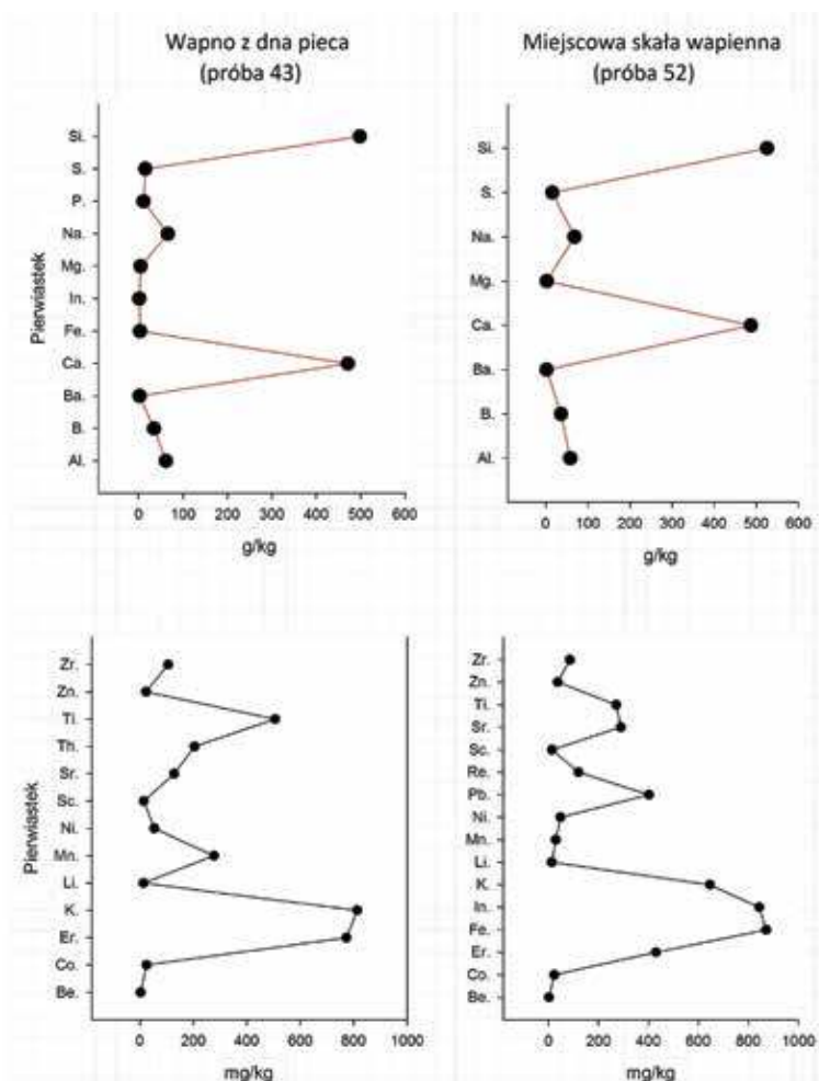
Ryc. 31. Wyniki analizy pierwiastkowej prób z wapiennika w Zimnochach, st. 2 (oprac. M. Sierakowski, oprac. graficzne F. Welc)
