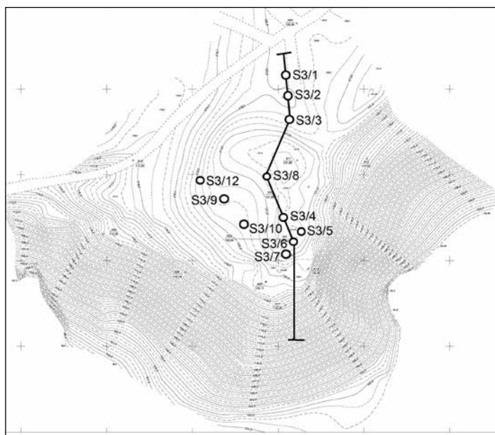
Ryc. 8. Plan warstwiczny grodziska w Zimnochach, st. 2 (wyk. J. Błaszczyk) z zaznaczonymi miejscami wierceń geologicznych (oprac. J. Nitychoruk i F. Welc)
