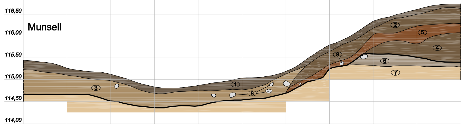
Ryc. 11. Plichta, st. 1. Plan wykopu 1 na poziomie warstw związanych z Fazą I i II oraz ściana północna wykopu 1 (oprac. R. Solecki i J. Wysocki)
