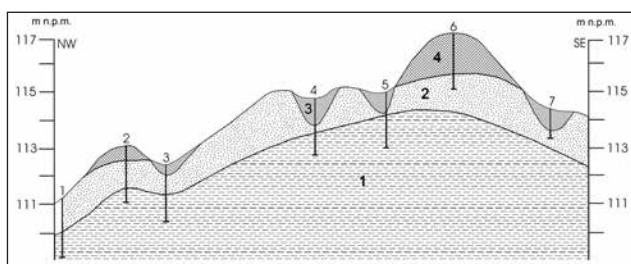
Ryc. 8. Przekrój geologiczny przez grodzisko w Plichcie, st. 1: 1 - mułki; 2 - piaski i piaski z mułkiem; 3 - piaski z organiką - wypełnisko fos; 4 - piaszczyste nasypy wałów (oprac. J. Nitychoruk i F. Welc)
