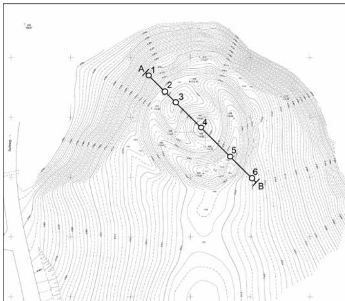
Ryc. 7. Plan warstwicowy grodziska w Plichcie, st. 1 (wyk. J. Błaszczyk) z zaznaczonymi miejscami wierceń geologicznych (oprac. J. Nitychoruk i F. Welc)
