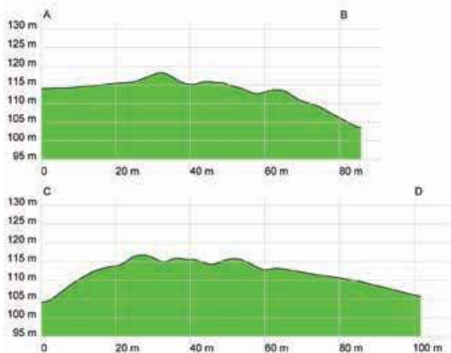
Ryc. 6. Przekrój grodziska w Plichcie, st. 1 po osi zbliżonej do północ-południe (A-B) i osi zbliżonej do wschód-zachód (C-D) uzyskany z danych ALS (na podstawie materiałów CODGiK, oprac. R. Solecki)
