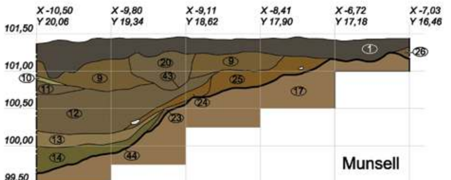
Ryc. 12. Laseczno Małe, st. 1. Przekroje przez nawarstwienia związane z użytkowaniem kopca (oprac. M. Rutyna, J. Wysocki i R. Solecki)
