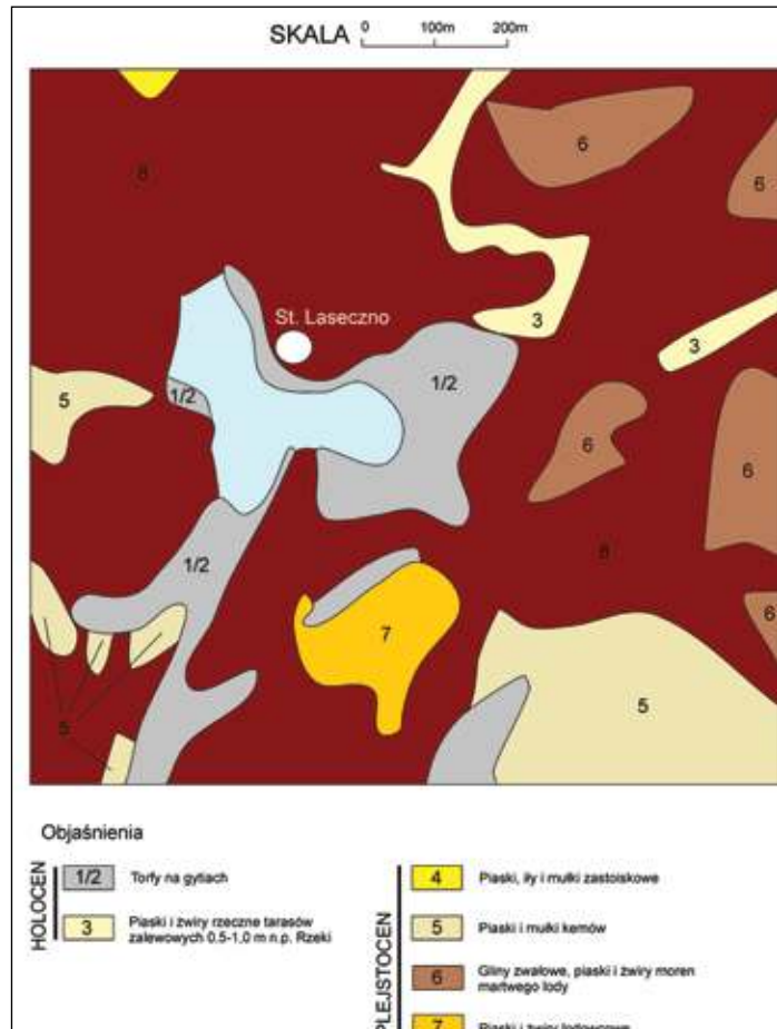
Ryc. 6. Mapa geologiczna okolic grodziska w Lasecznie Małym, st. 1 (oprac. J. Nitychoruk i F. Welc)
