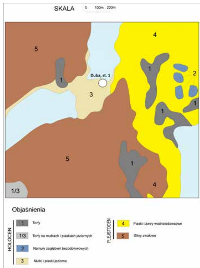
Ryc. 11. Mapa geologiczna okolic grodziska w Dubie, st. 1 (oprac. J. Nitychoruk i F. Welc)
