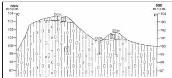
Ryc. 13. Przekrój geologiczny przez grodzisko w Dubie, st. 1: 1 - glina zwałowa, 2 - glina redeponowana, 3 - piasek drobnoziarnisty, wypełnisko fosi (oprac. J. Nitychoruk i F. Welc)
